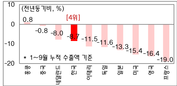
세계 10대 수출국의 '20.1~9월 수출
